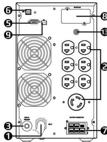
NEMA Type
