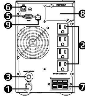
NEMA Type
