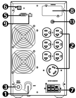
NEMA Type
